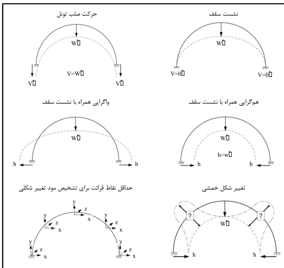
شکل ۴-۴- حالات مختلف تغییر شکل تونل
