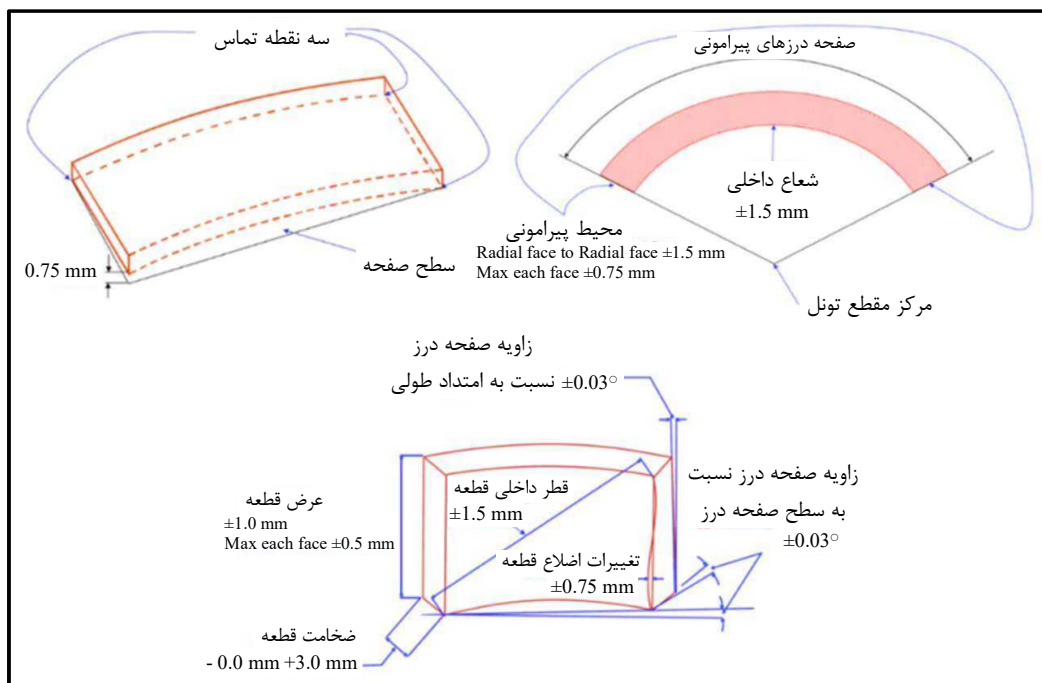
شکل ۶-۴- رواداری‌های ساخت و نصب سگمنت
