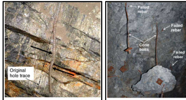
شکل ۳-۲۰- گسیختگی گوه مانند و برشی پیچ سنگ
