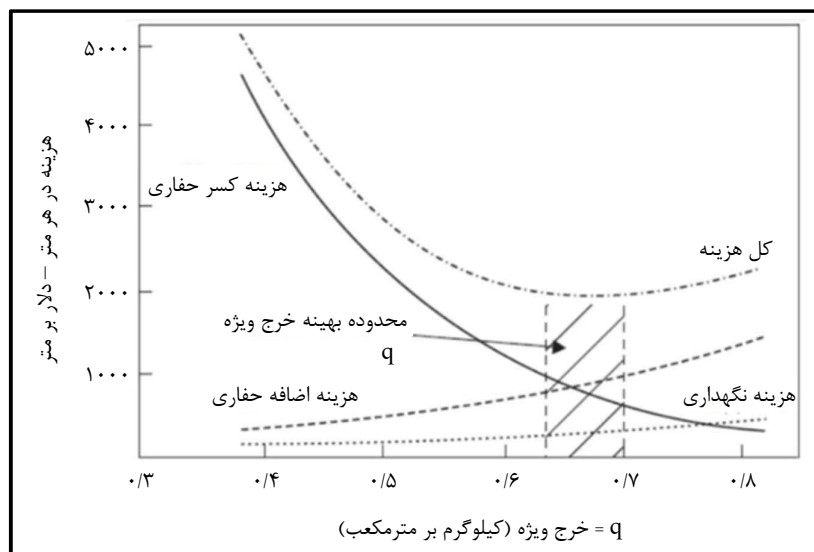
شکل ۳-۱- نمونه بهینه‌سازی مقدار خرج ویژه براساس سرعت پیشروی و هزینه‌های نگهداری و اضافه حفاری
