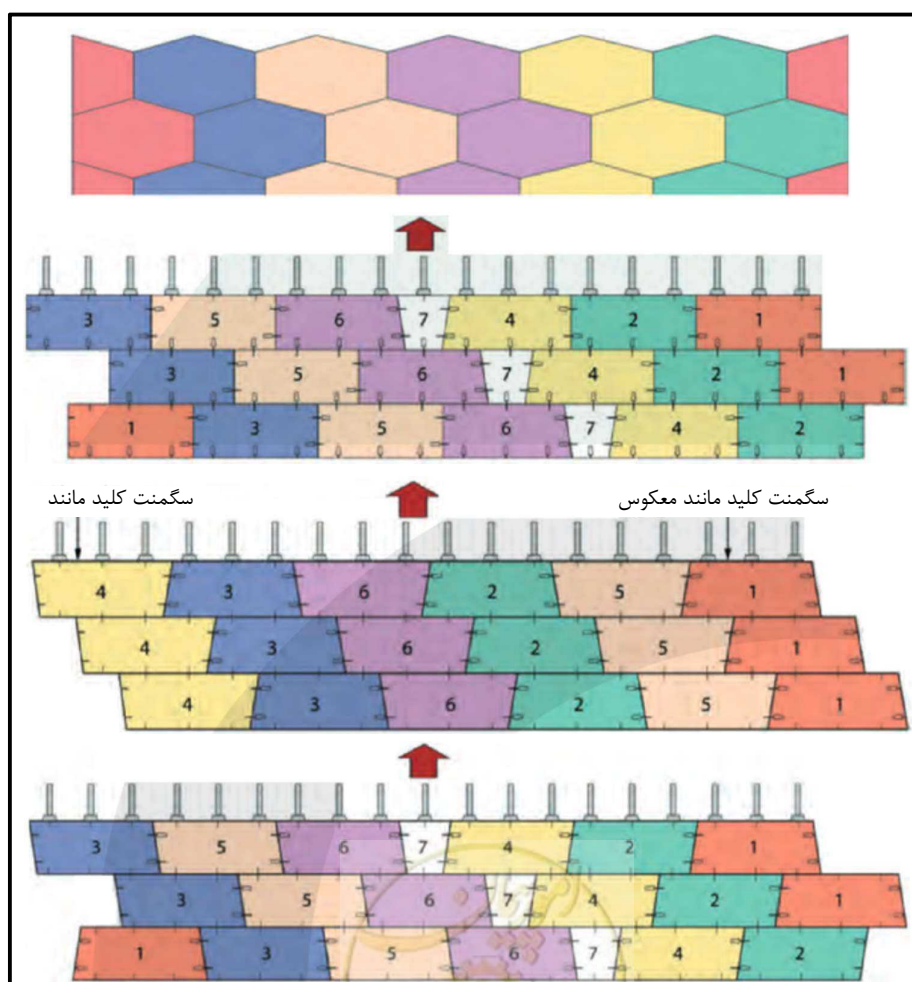
شکل ۶-۱۰- نقشه نصب انواع سگمنت شش ضلعی، مستطیلی با قطعه کلید، دوزنقه‌ای کلید مانند، متوازی‌الاضلاع با قطعه کلید
