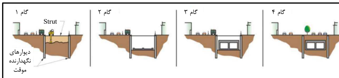
شکل ۲-۲- روش اجرای کندوپوش پایین به بالا
