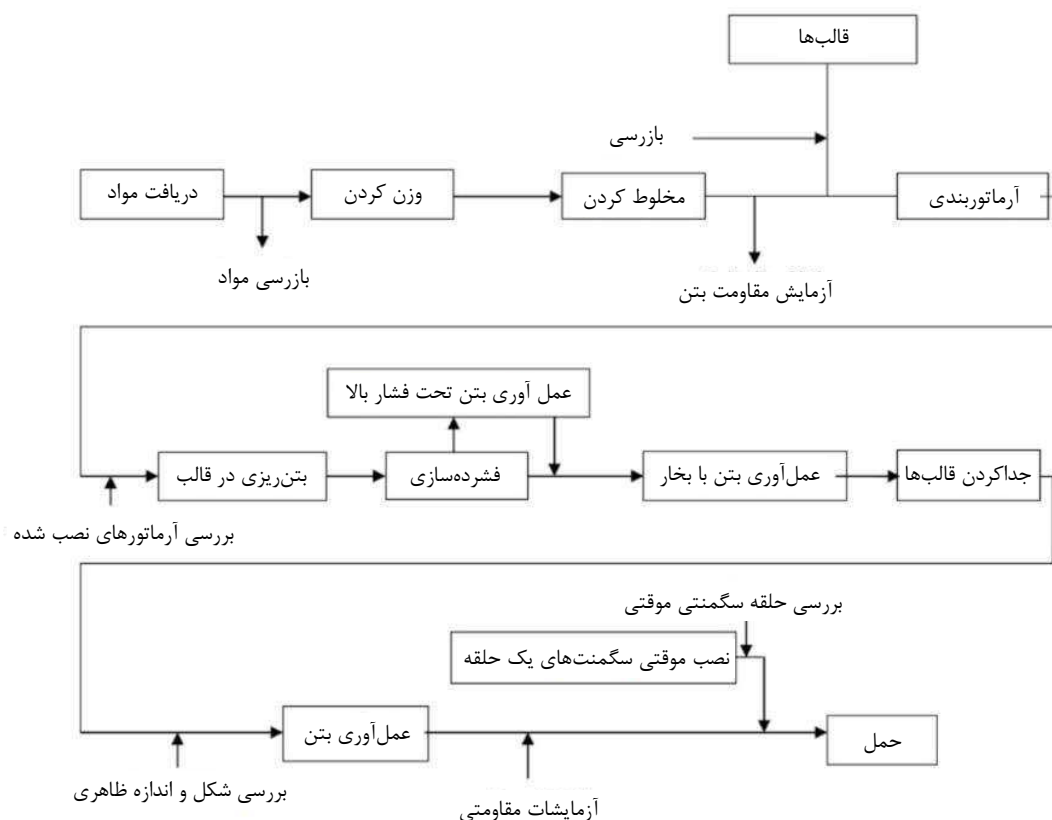
شکل ۵-۱۴- دیاگرام فرآیند تولید قطعات پیش‌ساخته پوشش تونل
