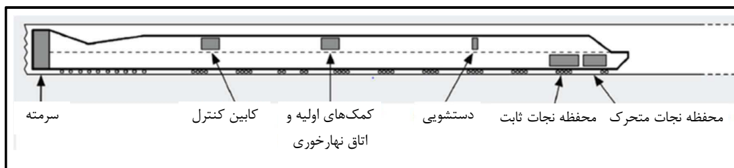
شکل ۷-۳- جانمایی اتاق امن و نجات در انتهای ماشین حفاری مکانیزه تونل
